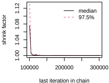
d.Erlotinib.DHFRi
