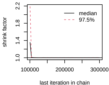
d.Osimertinib.Lazertinib
