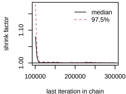
d.Erlotinib.Erlotinib_HER3i
