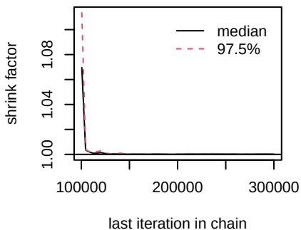
d.Gefitinib_Erlotinib.Zorifertinib
