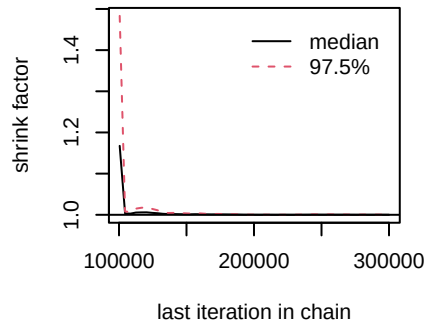
d.Erlotinib.Rociletinib
