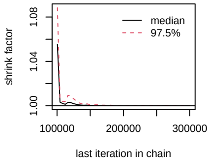
d.Erlotinib.Erlotinib_METi
